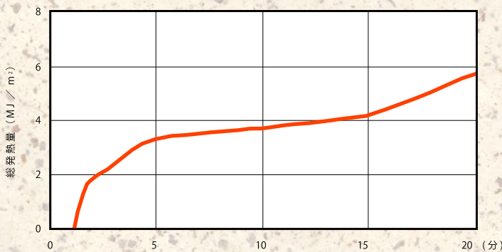
コーンカロリメーターによる発熱性試験
