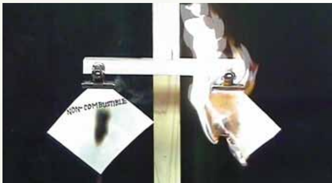
不燃和紙の燃焼実験（左：セルフネン液含浸処理、右：処理なし）
